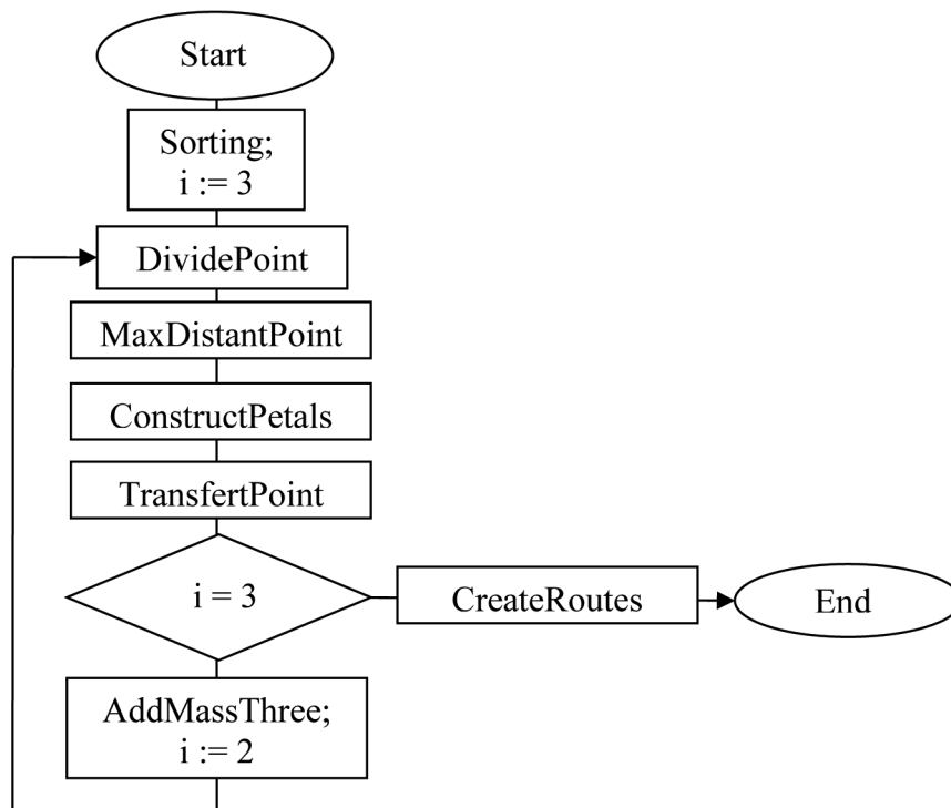
Рис.1 Блок-схема работы алгоритма
