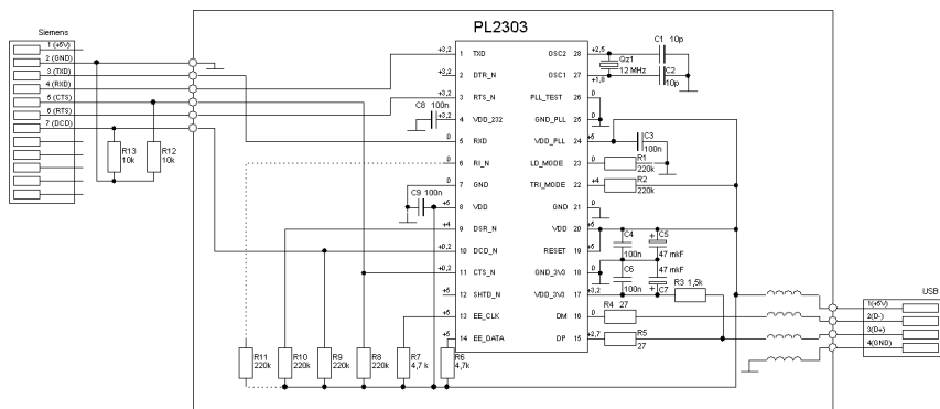
Рисунок 2. Схема интерфейсного кабеля на микросхеме PL2303
