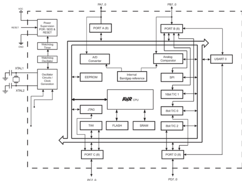
Рисунок 1. Блок-схема микроконтроллера ATmega644
