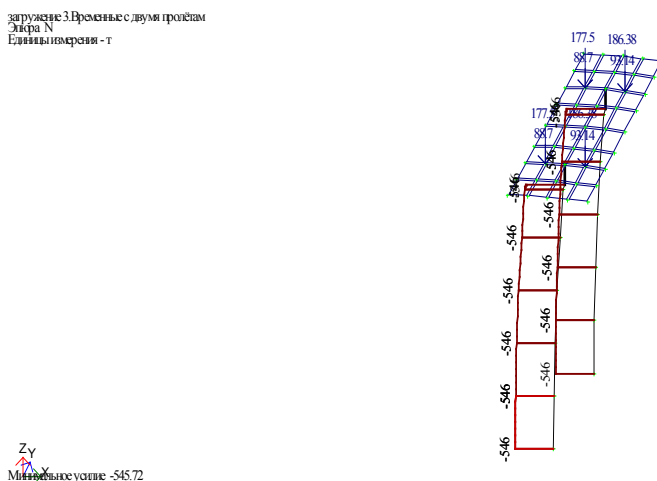
Рис 4. Эпюра по вертикальной нагрузке N
