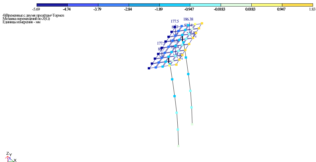
Рис 3. Деформированное состояние опоры (поперек моста) от данного сочетания нагрузок
