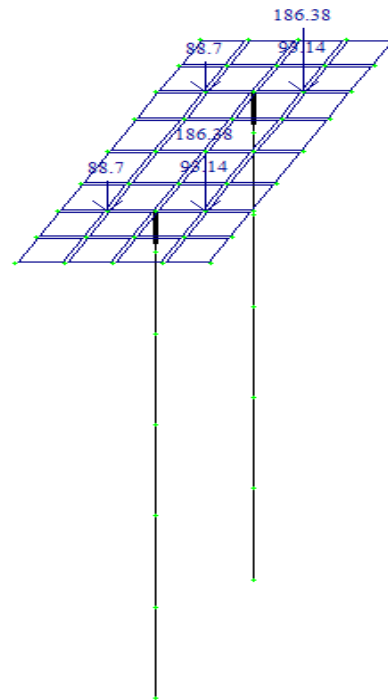
Рис. 2. Схема загрузки статических нагрузок промежуточной опоры железнодорожного моста:
